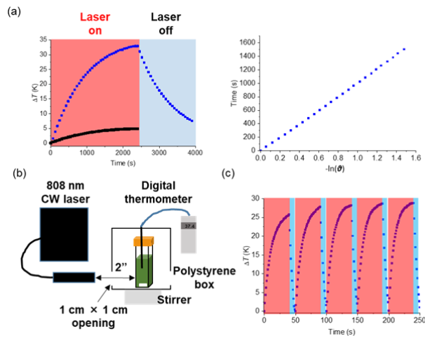
図 2. P の光熱効果。(a) V-NC (青)と、水 (黒)をドーピングした P ドットの温度変化。(b) 光熱効果実験の模式図。(c)V-NC をドーピングした P-dots の温度変化に対する安定性テスト。(研究成果の論文より転載)。
