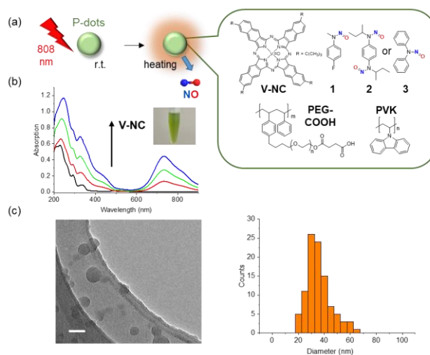
図 1. (a) 808 nm の NIR 光照射による NO と熱放出の模式図。(b) V-NC をドーピングした P-dots の吸収スペクトル。(c) TEM 画像と直径の分布を示すヒストグラム (研究成果の論文より転載)。
